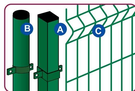
appoggiare il pannello C sul montante A o B
