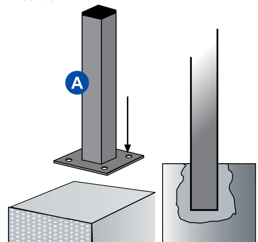
con piastra cementato Sistemi di Fissaggio del montante.
