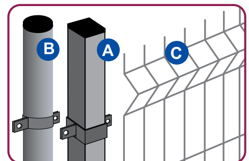
appoggiare il pannello C sul montante A o B
