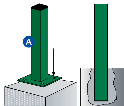
con piastra cementato Sistemi di Fissaggio del montante.
